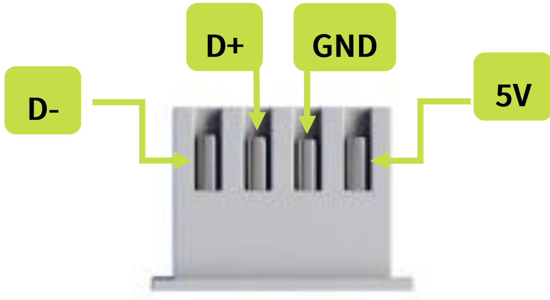
USB 端口线序
